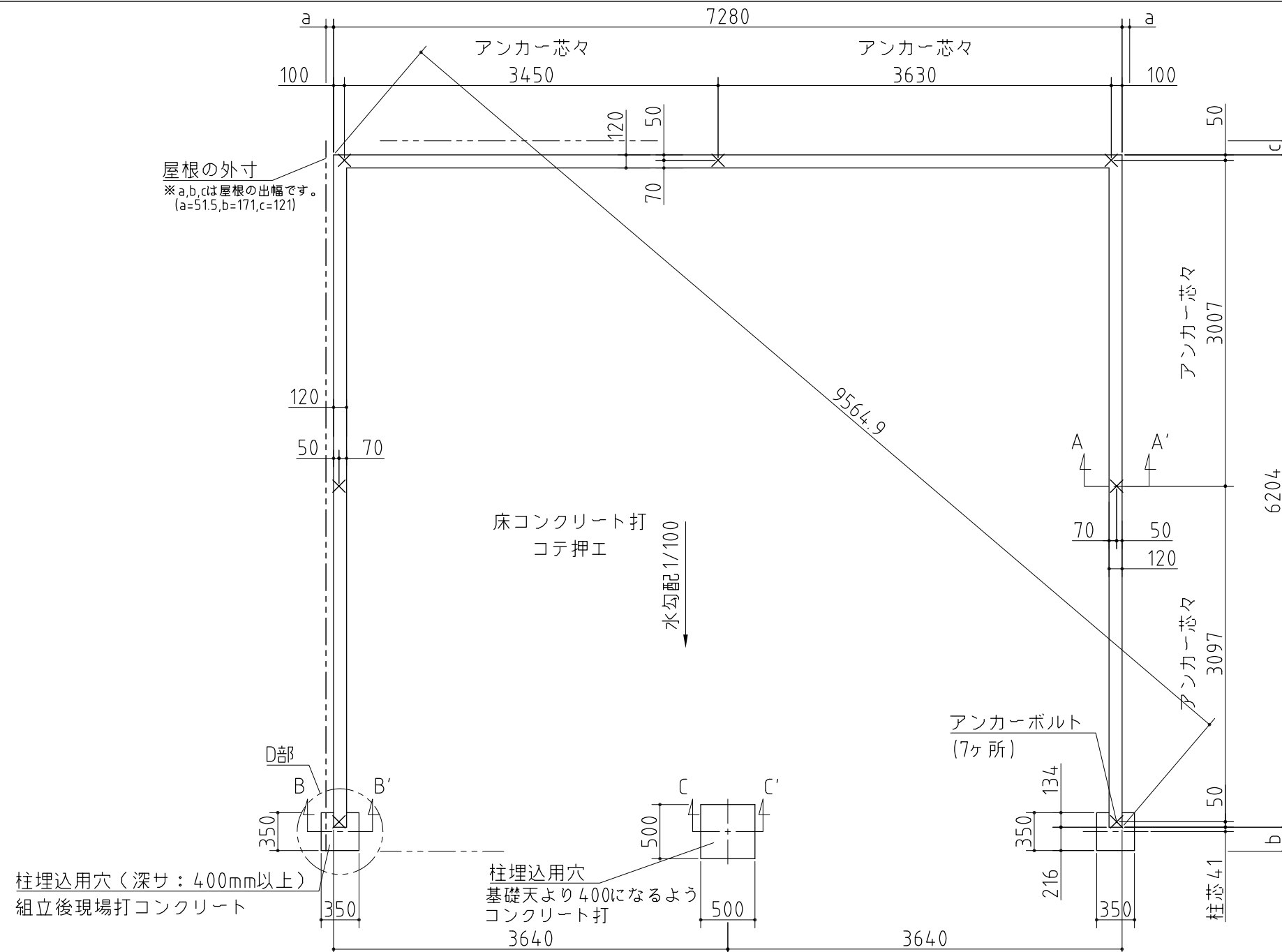
基礎詳細図 S=1/20
